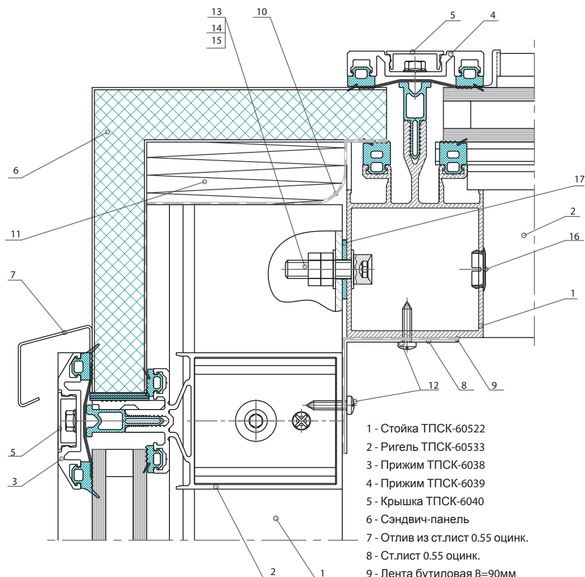
1-1 ИСПОЛНЕНИЕ 1
