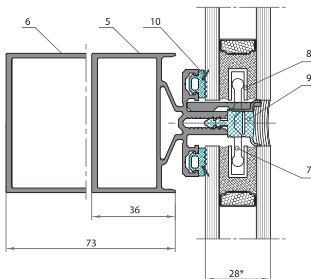
3 ИСПОЛНЕНИЕ 2
