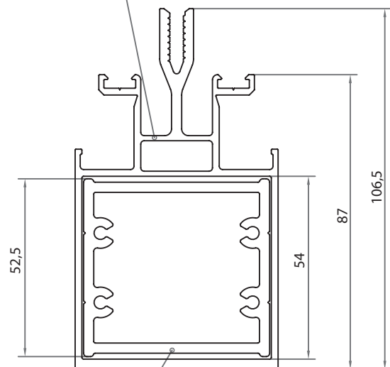
ТПСК-60512
