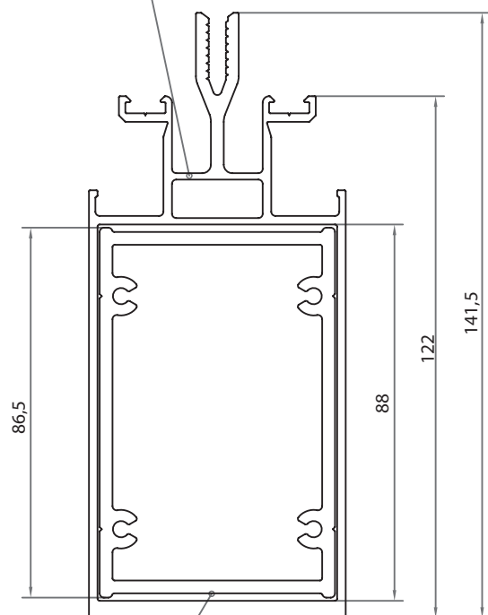
ТПСК-60513
