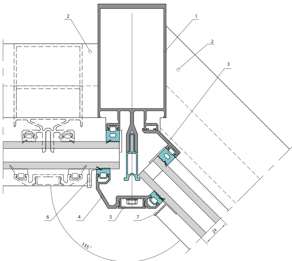
1 (ВНУТРЕННИЙ УГОЛ 135°)
